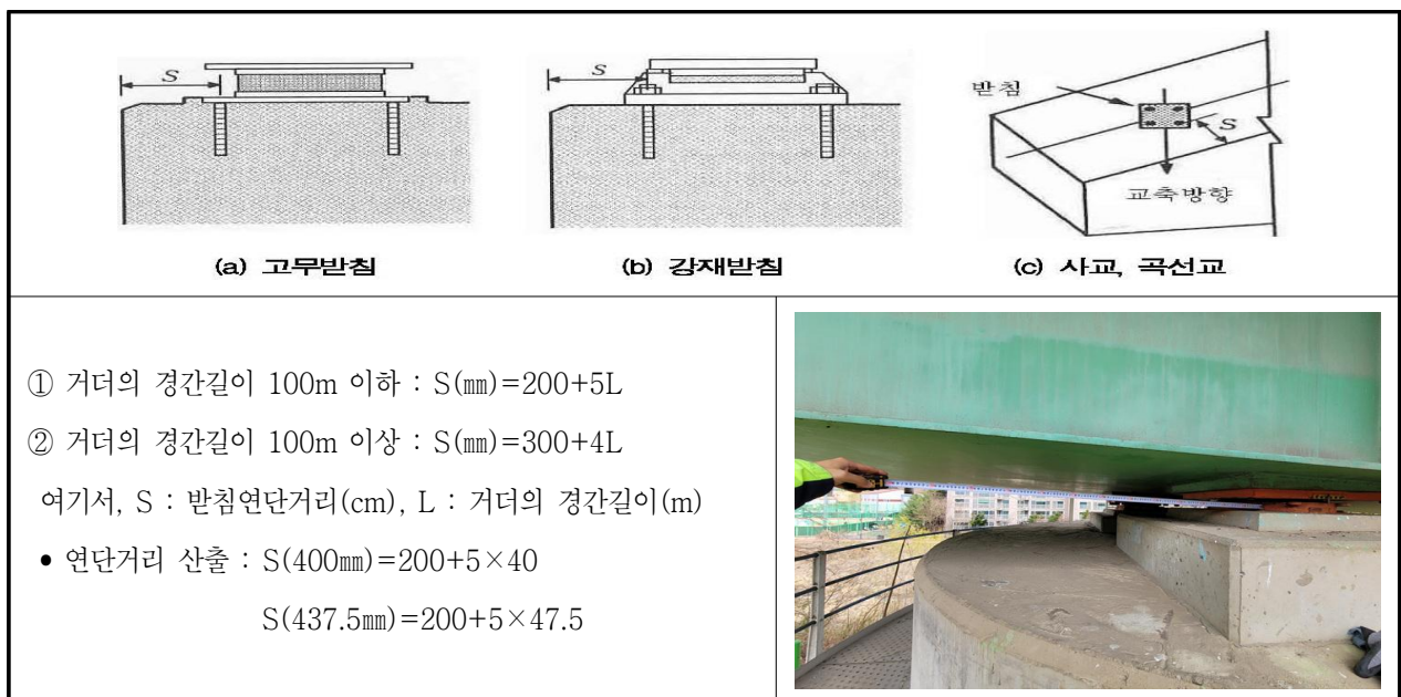
【그림 1.3.2】 도로교설계기준 연단거리 산출방법
