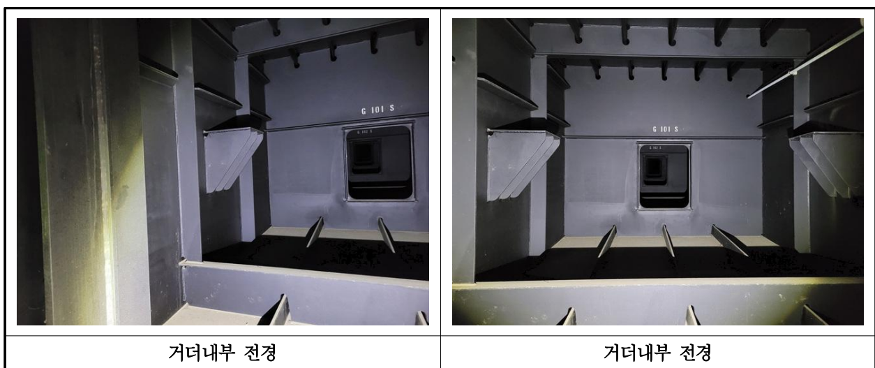
【사진 1.3.6】 거더내부 전경
