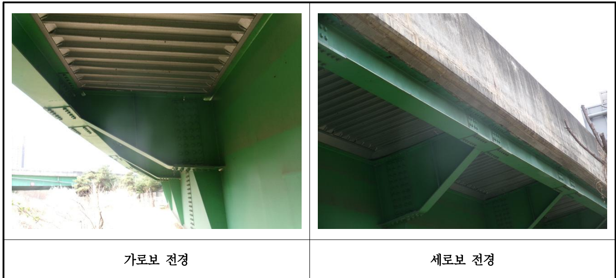
【사진 1.3.8】 가로보 및 세로보 전경
