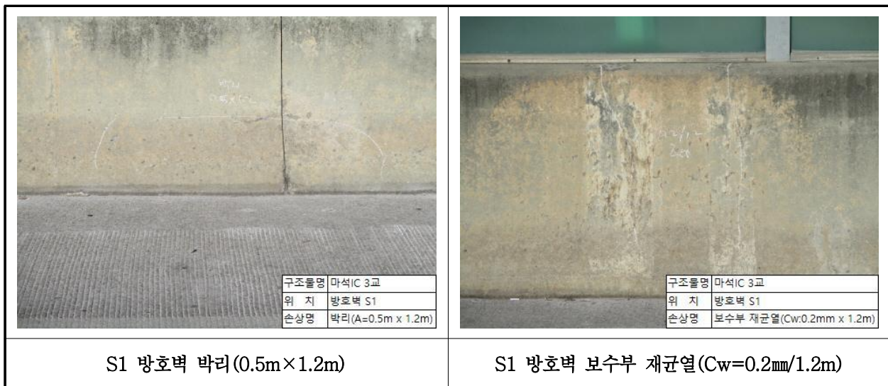
【사진 1.3.24】 방호벽 손상현황
