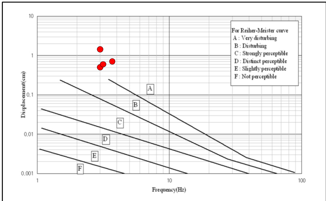
【그림 1.7.1】 Reiher-Meister(1931)의 허용곡선
