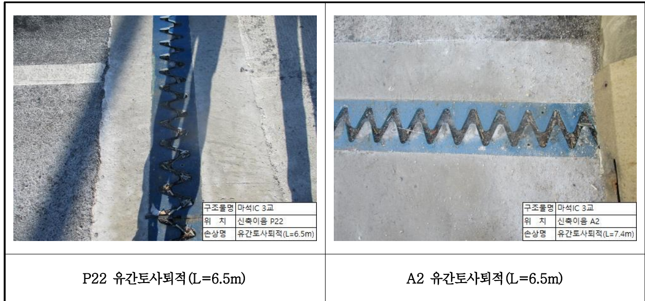
【사진 1.3.17】 신축이음장치 손상현황
